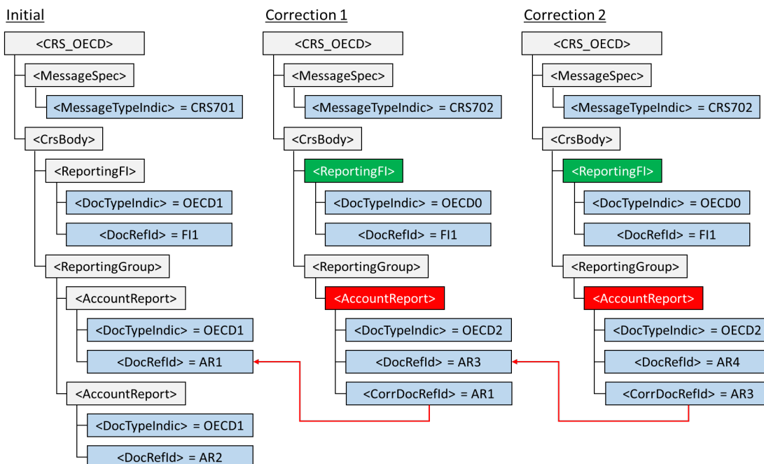
Abbildung 2: Zweimalige Korrektur eines AccountReports nach CRS-XML-Schema
