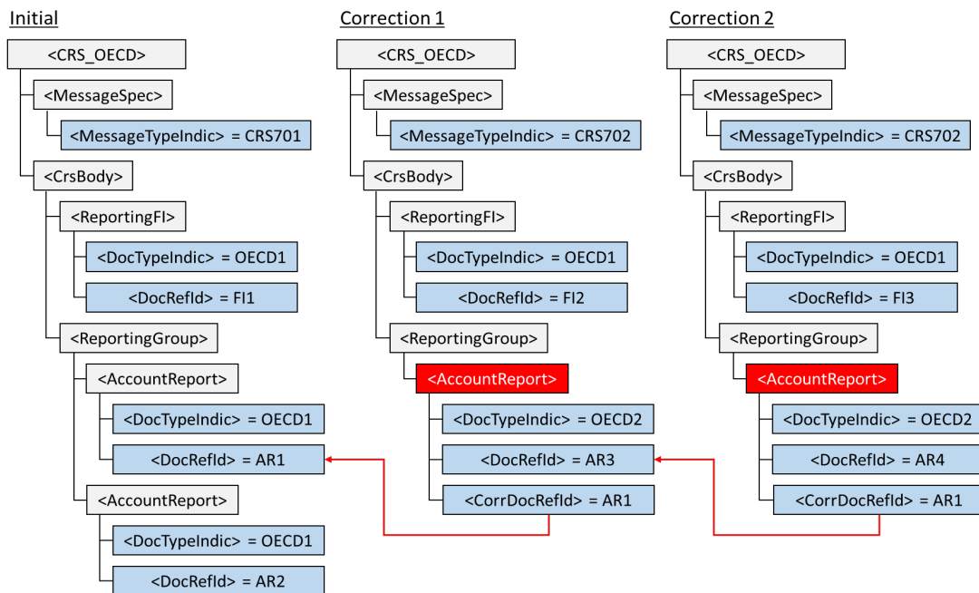
Abbildung 3: Zweimalige Korrektur eines AccountReports alternativ
